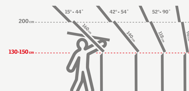
Krovni prozori sa središnjim vješanjem krila
