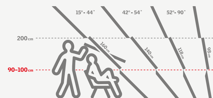
Krovni prozori sa središnjim vješanjem krila
