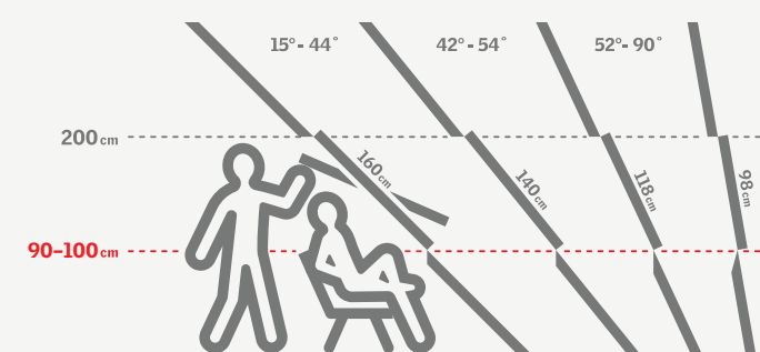
Sredinsko vpeto strešno okno z ročico zgoraj.
