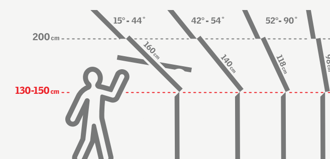
Sredinsko vpeto strešno okno z ročico zgoraj.
