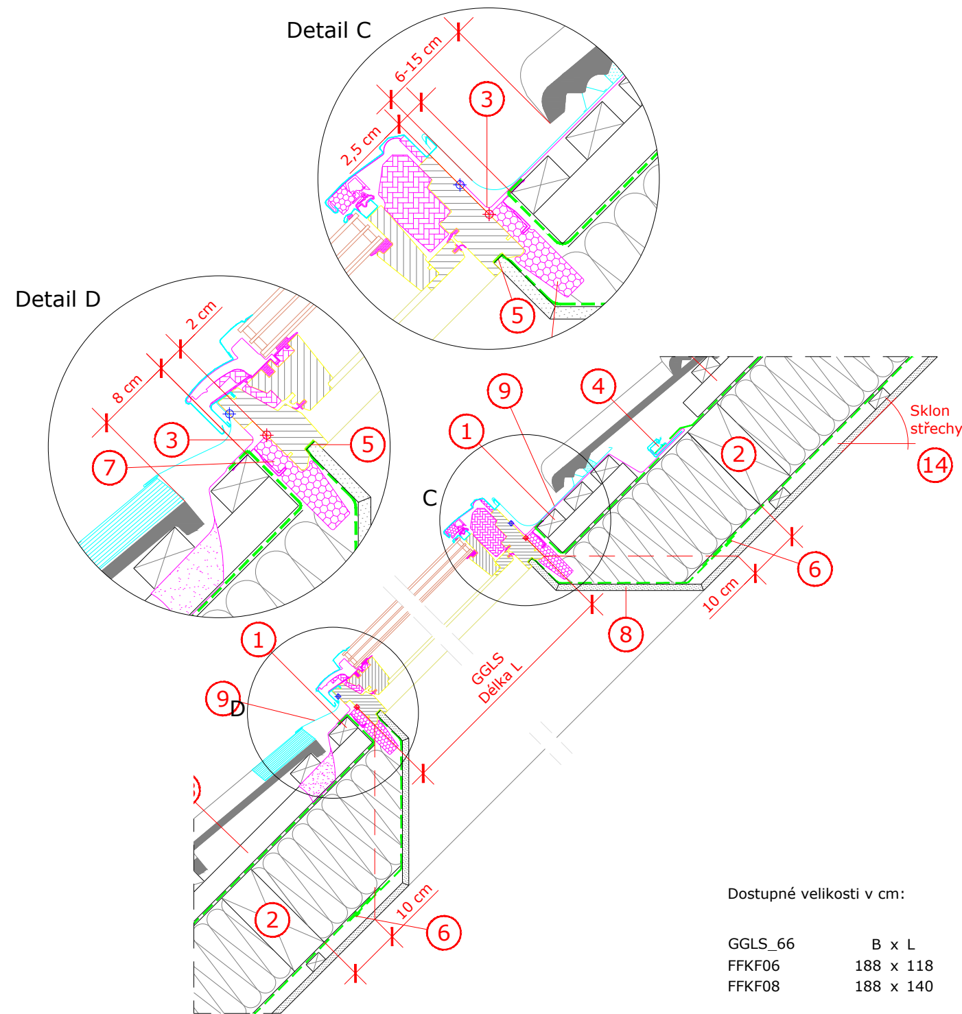
Řez B - B, fixní středový díl
