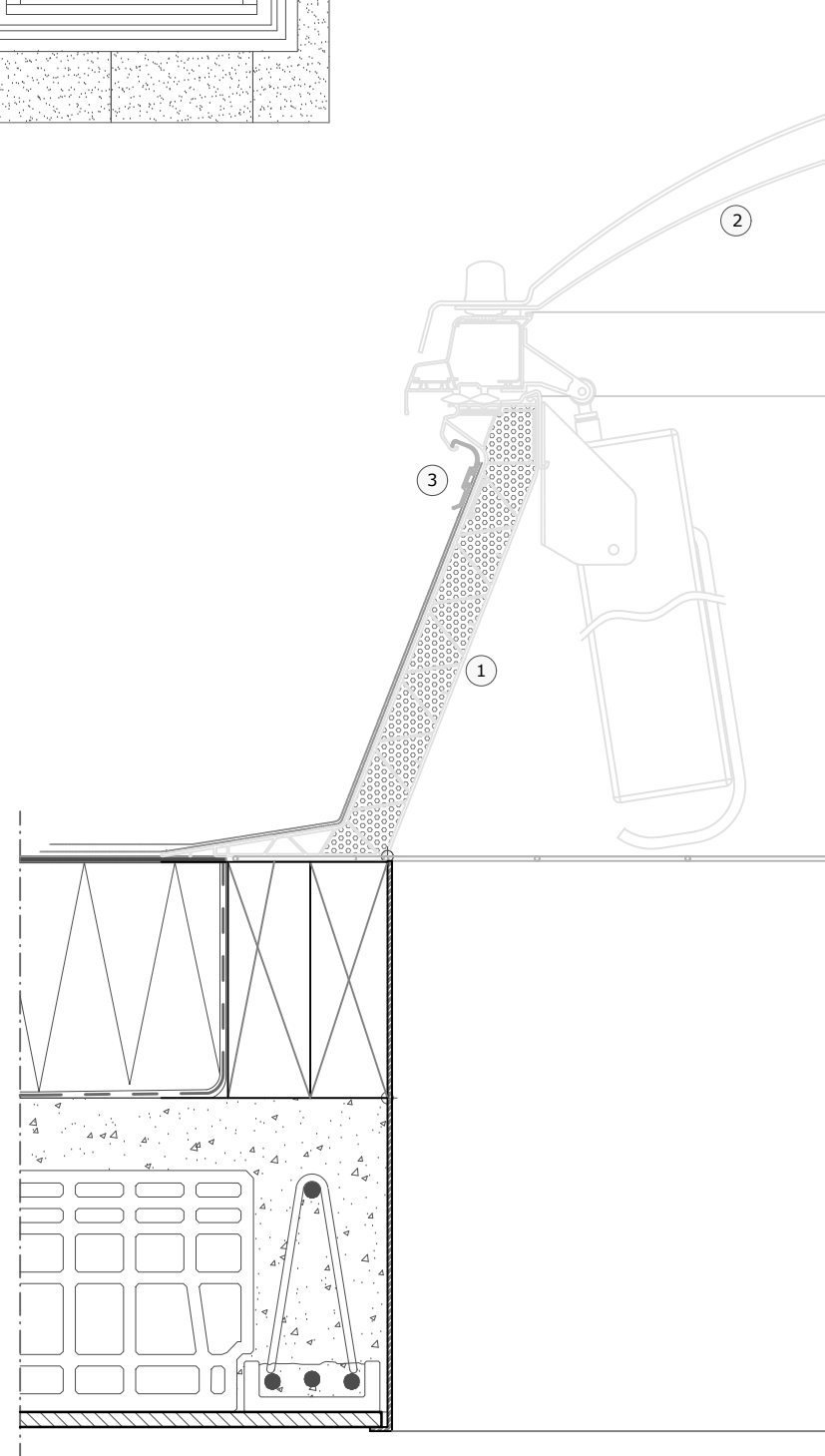
Sectiune A-A 1:5
