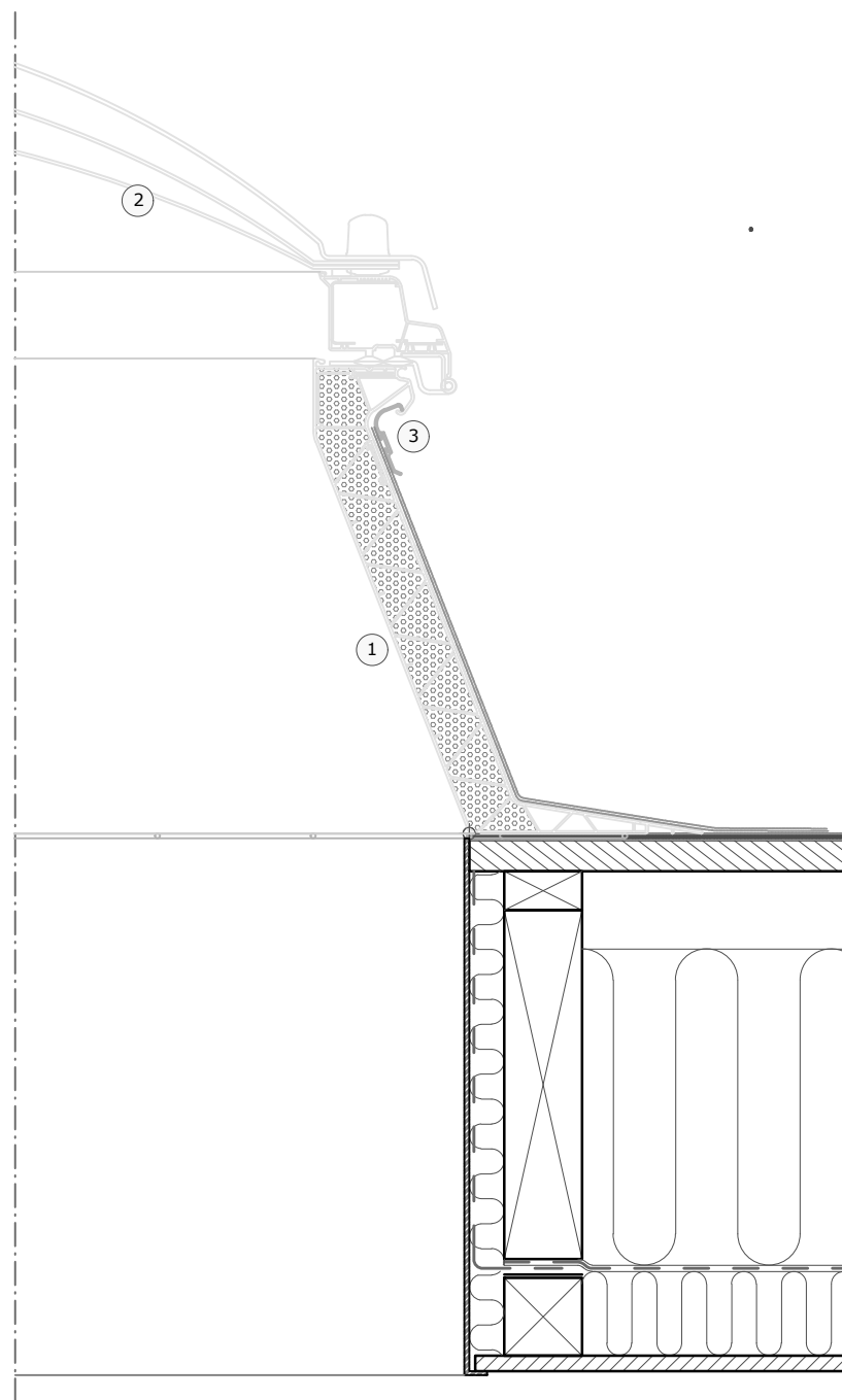
Sectiune A-A 1:5
